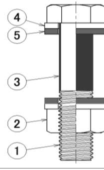
タイプVSⅡ 材料表 (1組当たり)
