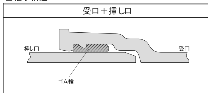
■継手構造
