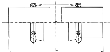
CL-A型 (250mm以下)
