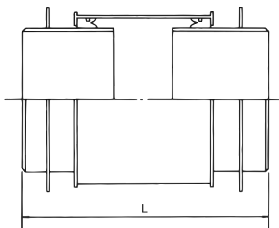
両ベベル形
