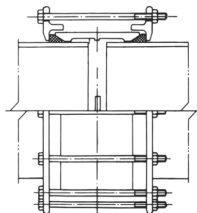
D型1000A以上
