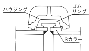
S—1 型 (2.0MPa 用)
