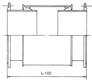
両フランジ形
