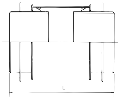
両ベベル形
