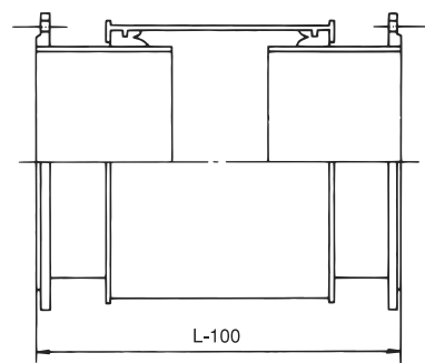
両フランジ形
